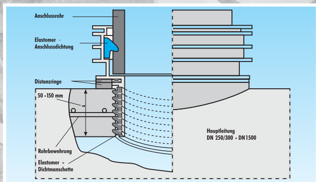
schematische Darstellung des Bohranschlussstutzens
